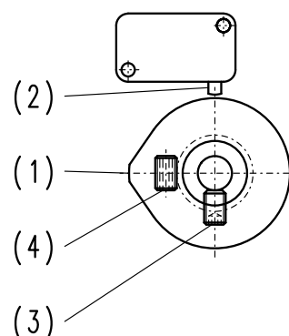
Fig. 1: Eindschakelnok
