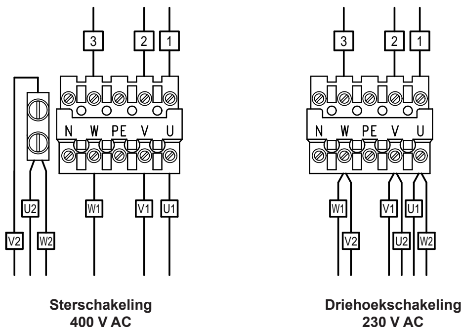
Fig. 1: Motorstekker met stekverbinding
