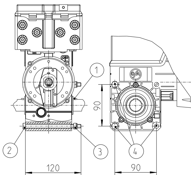
Fig. 1: Opsteekbare aandrijving
