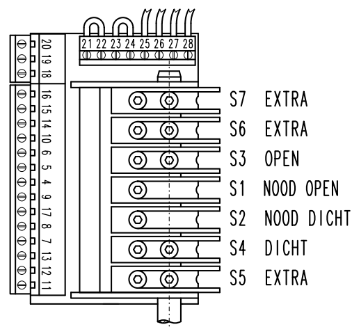
Fig. 2: Printplaat
