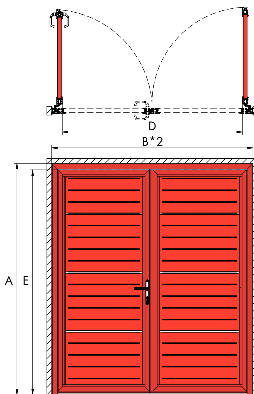
Montage in de dag met afdeklijst buiten
